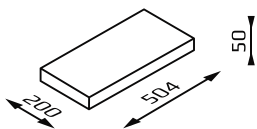
CH20, CRP20, CRD20 Pfeilerabdeckung / Mauerabdeckung
