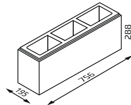
RM19 Pfeilerblock / Mauerblock
