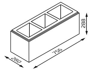
RM28 Pfeilerblock / Mauerblock
