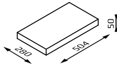
CH28 Pfeilerabdeckung / Mauerabdeckung
